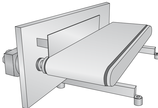
SWB-300 Open Frame (belt width 300mm)
